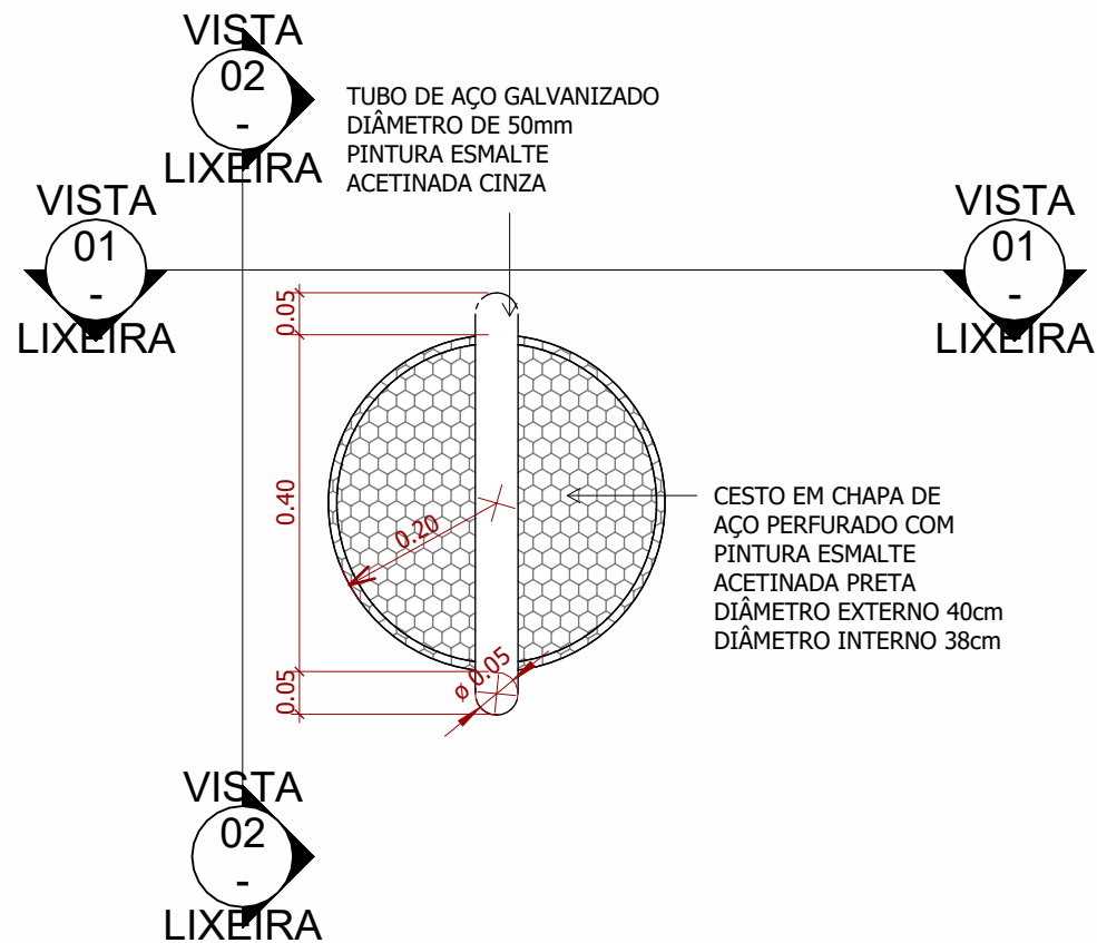
1 PLANTA BAIXA - LIXEIRA ESC.: 1 : 10
